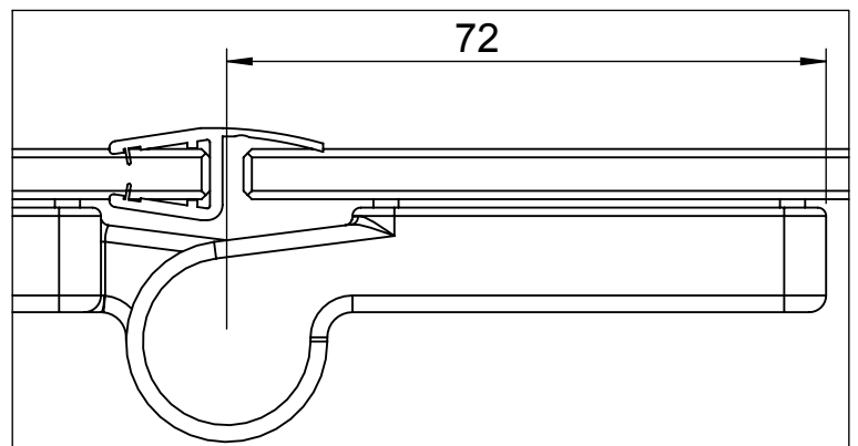
DETAIL B 1 : 1
