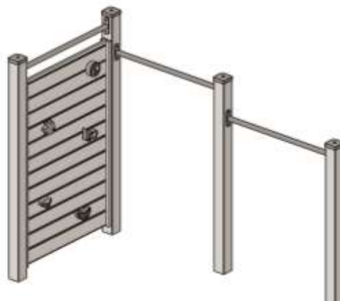
Aufbauvariante 2
