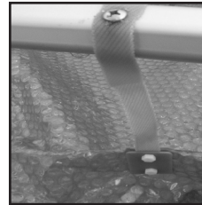
Fixez la sangle sur le tube en aluminium à l'aide d'une des vis 6 x 20 mm après avoir effectué le pré-perçage
