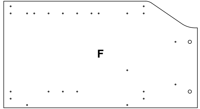
866x480x18mm
