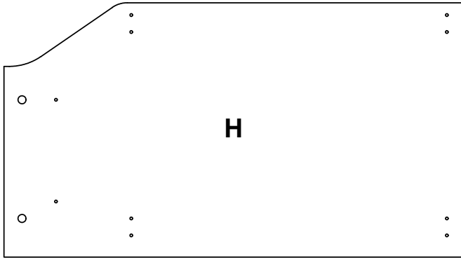
866x480x18mm
