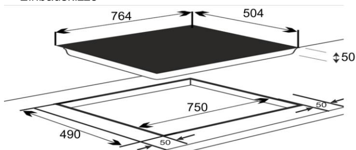
Einbauskizze
