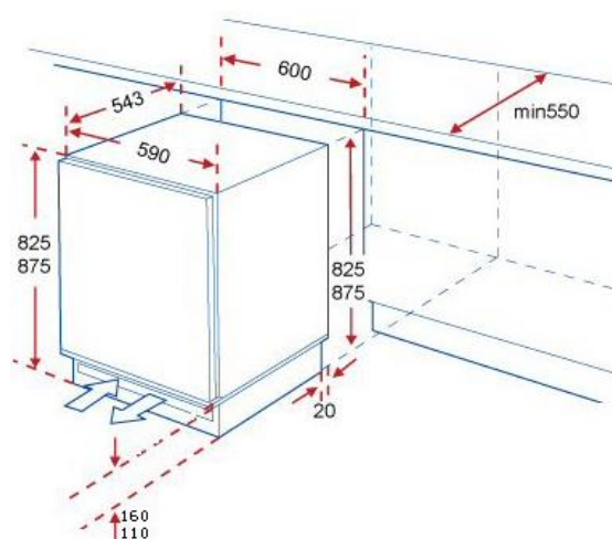
Einbauskeizze
