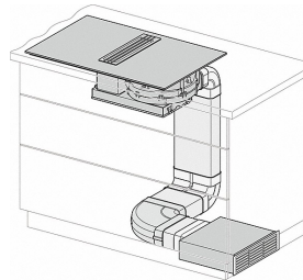
KMDA 7774, Einbauvariante 1 (Skizze)
