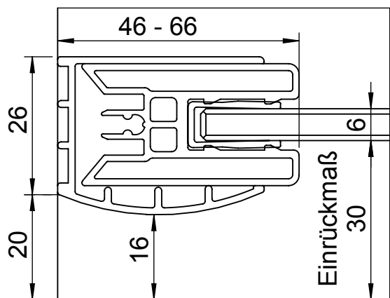
DETAIL A 1 : 1
