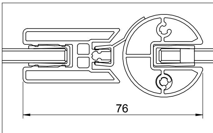
DETAIL B 1 : 1
