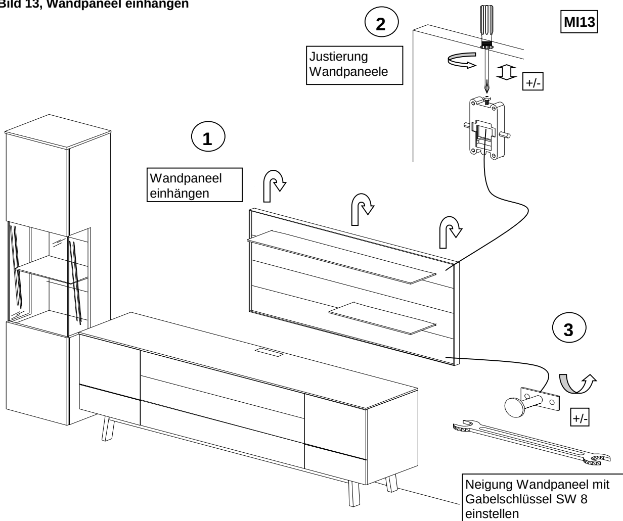
Bild 13, Wandpaneel einhängen
