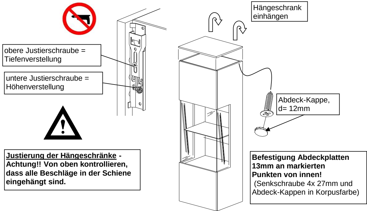
Bild 5, Hängeschränk einhängen, Abdeckplatte befestigen
