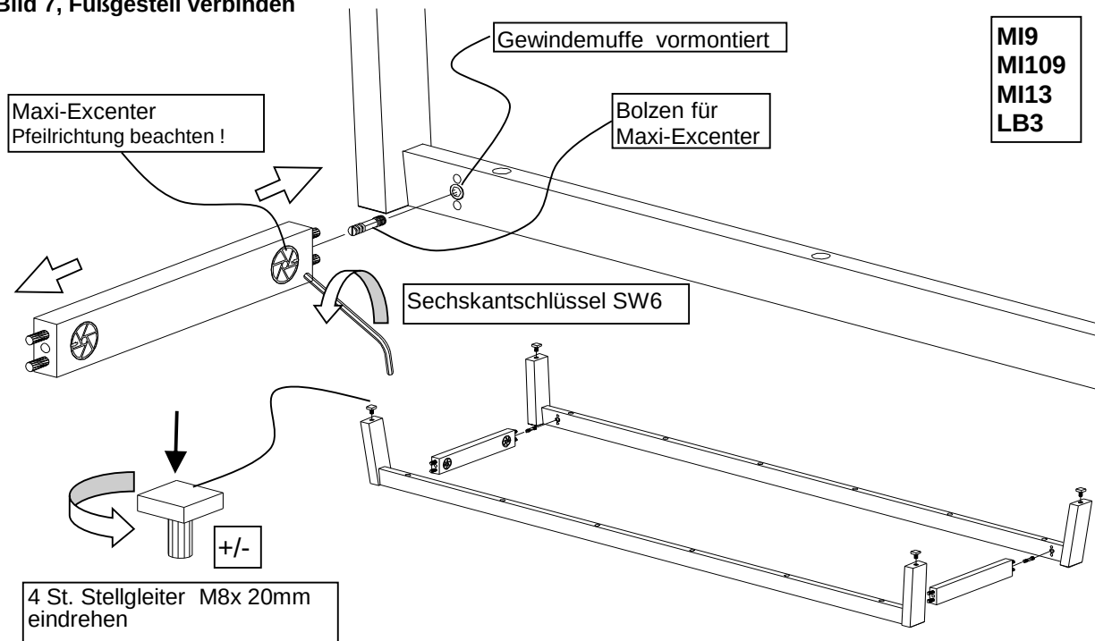
Bild 8, Fußgestell befestigen
