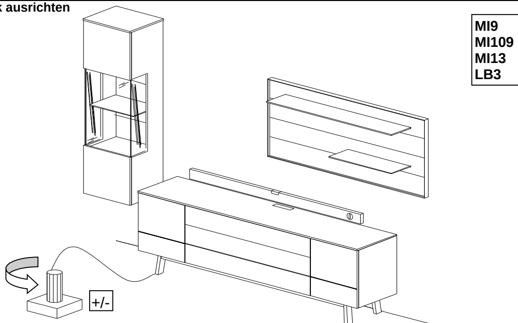
Bild 9, Schrank ausrichten
