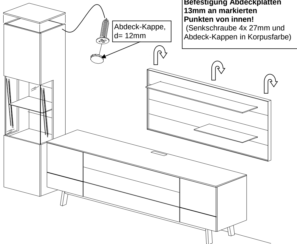
Bild 12, Abdeckplatte befestigen
