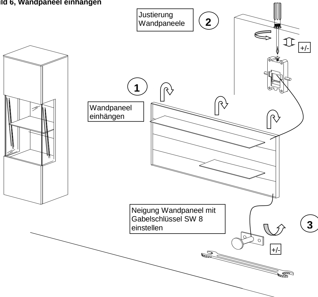
Bild 6, Wandpaneel einhängen
