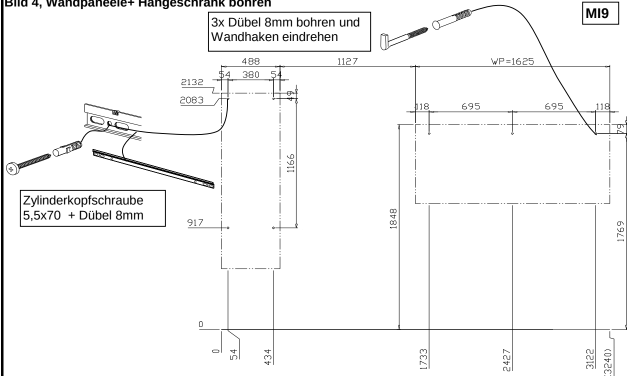
Bild 4, Wandpaneele+ Hängeschränk bohren
