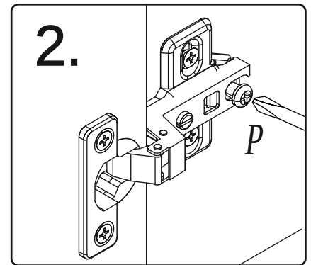
Türverstellungsschema (falls erforderlich) Door adjustment scheme (if necessary)
