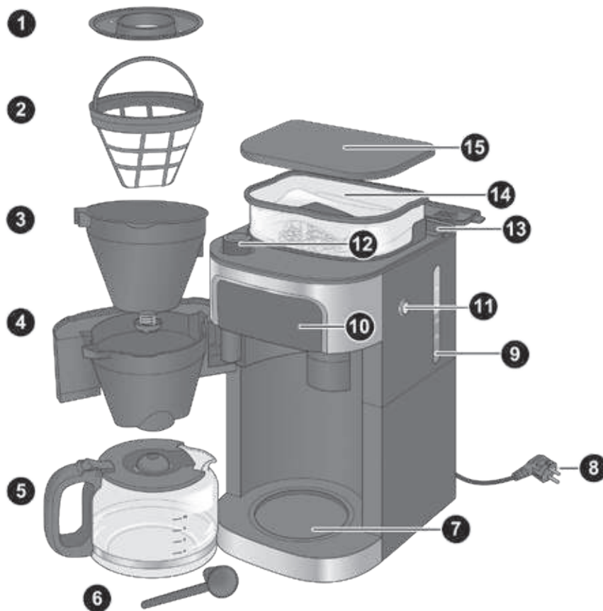
Bild 1: Apparatsens delar
