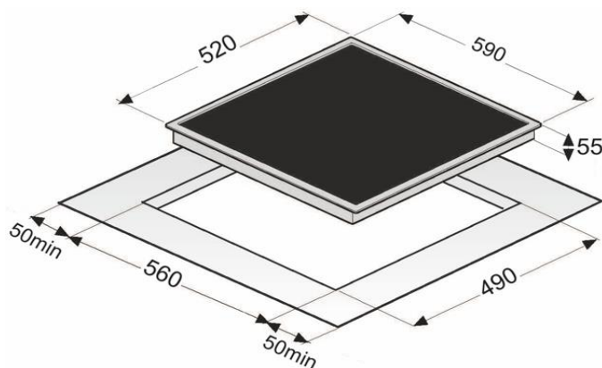
Einbauskizze
