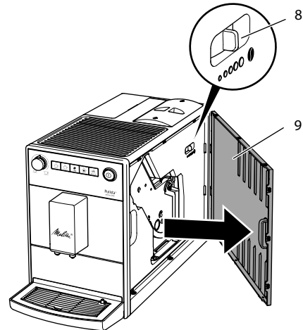
Abb. 11: Mahlgrad einstellen
