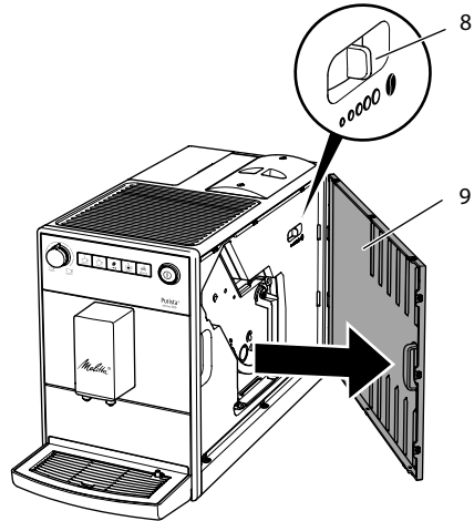
Afb. 11: Maalgraad instellen
