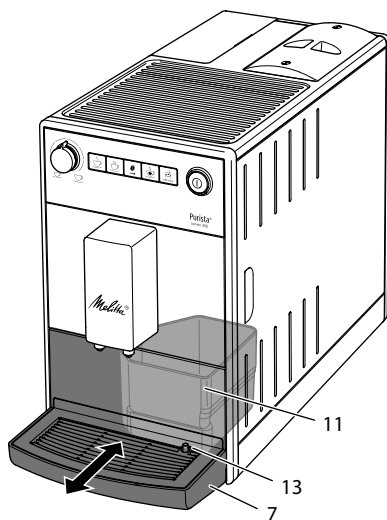
Bild 8: Tömma droppskålen och behållaren för kaffesump
