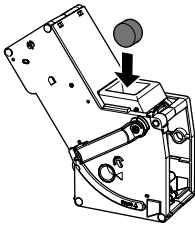
Pav. 14: Valymo tabletės įdėjimas į plikymo bloką.
