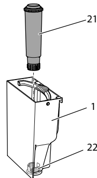
Fig. 15: Montaggio e smontaggio del filtro dell'acqua
