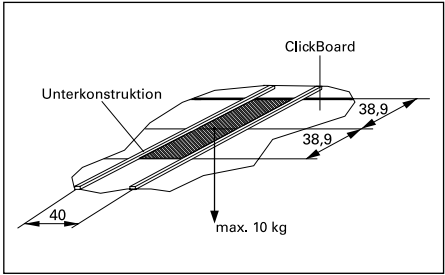
Zulässige Belastung pro Deckenflächeneinheit (40 cm × 77,8 cm (2 × 38,9 cm))
