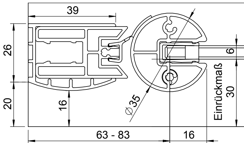
DETAIL A 1 : 1
