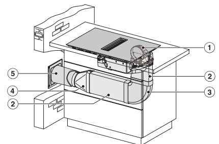
KMDA7272FL/FR, KMDA7473FL/FR – Einbauvariante 9 Abluft – Skizze
